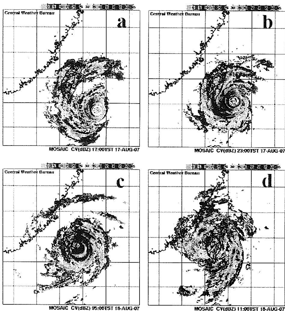
圖 7. 2007 年 8 月 (a) 17 日 0900 UTC、(b) 17 日 1500 UTC、(c) 17 日 2100 UTC、(d) 18 日 0300 UTC 之中央氣象局雷達網所觀測之雷達回波圖。
