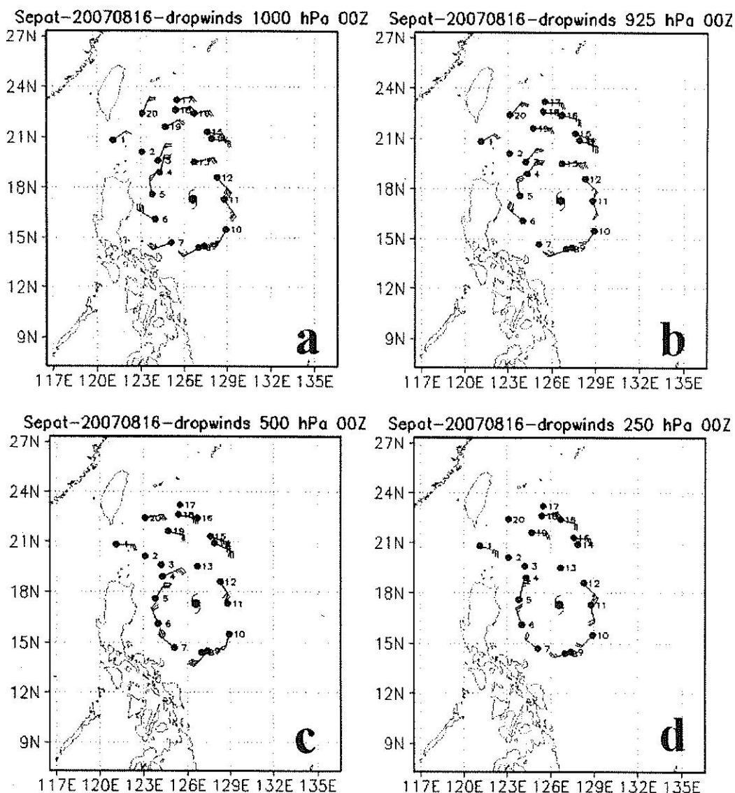
圖 6. 聖帕颱風 GPS dropwindsonde (a) 1000 hPa (b) 925 hPa (c) 500 hPa (d) 250 hPa 之觀測風場資料 (摘自台灣大學大氣科學研究所吳俊傑教授網站)。
