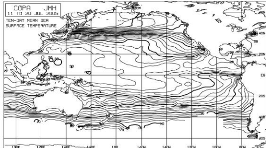
圖 9. 民國 94 年 7 月 11 日至 20 日 10 天平均海水溫度圖
