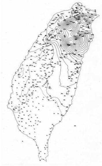
圖 13a. 海棠颱風日雨量分布圖(94 年 7 月 17 日零時至 24 時)
