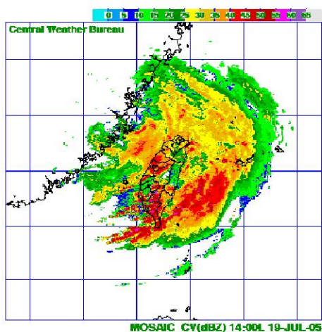
圖 12i. 同圖 12a, 但為 94 年 7 月 19 日 14 時 (地方時)
