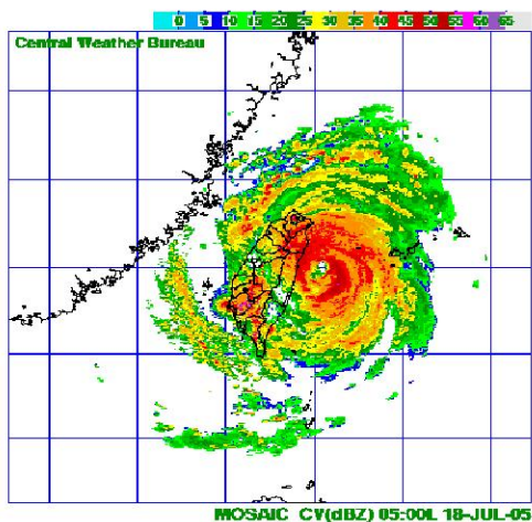
圖 12b. 同圖 12a, 但為 94 年 7 月 18 日 5 時(地方時) Fig. 12b. Same as 12a, but for 071805L 2005
