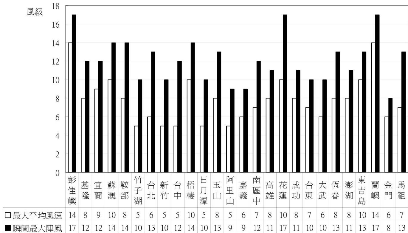
圖 11. 海棠颱風侵台期間各氣象站出現之最大風速與瞬間最大陣風(單位：級)
