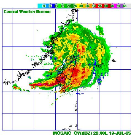
圖 12j. 同圖 12a, 但為 94 年 7 月 19 日 20 時 (地方時)
