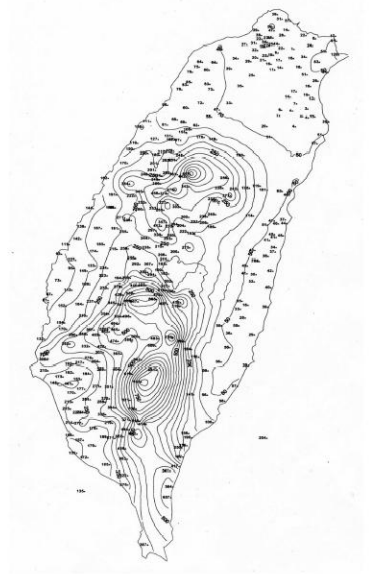
圖 13c. 海棠颱風日雨量分布圖(94 年 7 月 19 日零時至 24 時)
