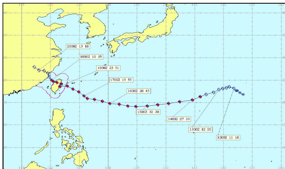
圖 1. 海棠颱風(0505)最佳路徑圖。圖中空心代表強度為輕度颱風，實心為中度以上颱風，標示資料由左至右分別為 UTC 時間(DDHH)、移速(km/hr)及近中心最大風速(m/s)。
