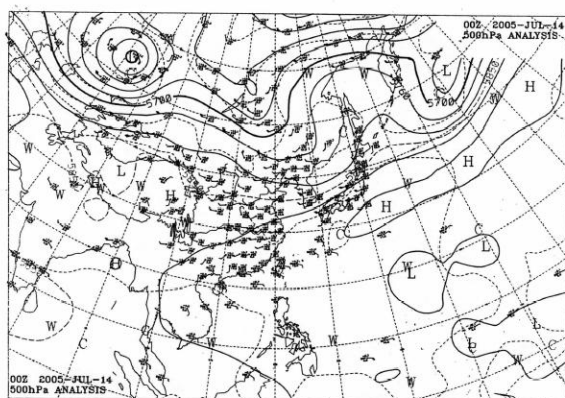
圖 2. 94 年 7 月 14 日 00UTC 500 百帕高空圖
