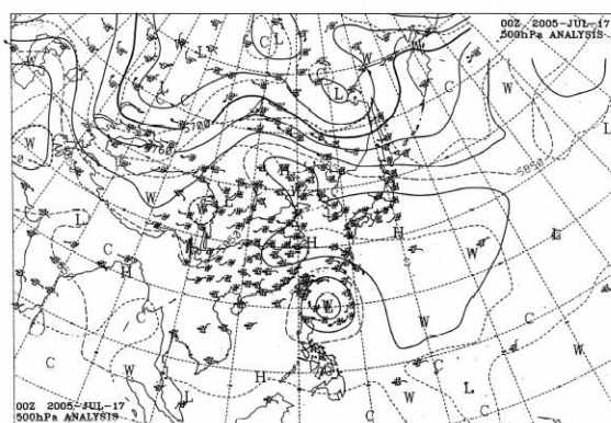
圖 5. 94 年 7 月 17 日 00UTC 500 百帕高空圖 Fig. 5. The 500hPa geopotential height and wind vectors at 00UTC July 17 of 2005
