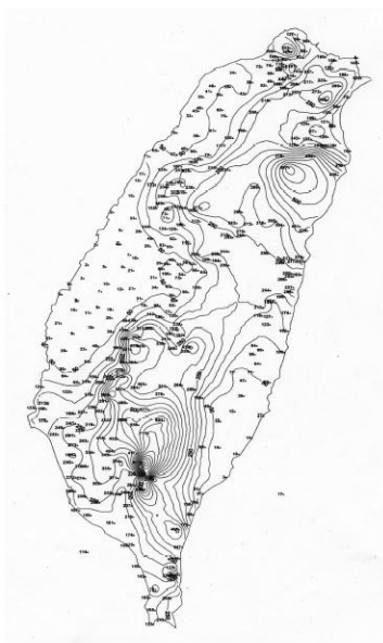
圖 13b. 海棠颱風日雨量分布圖(94 年 7 月 18 日零時至 24 時)
