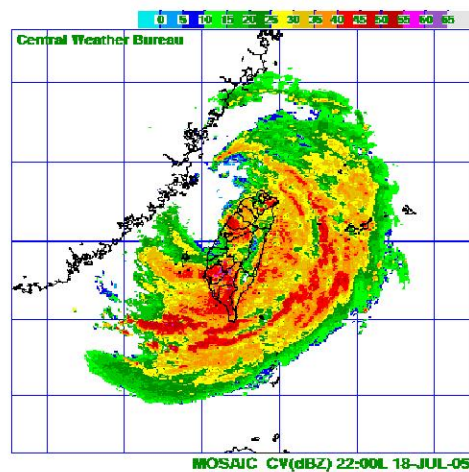
圖 12g. 同圖 12a, 但為 94 年 7 月 18 日 22 時 (地方時)
