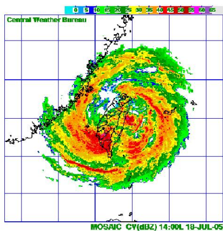
圖 12d. 同圖 12a, 但為 94 年 7 月 18 日 14 時(地方時) Fig. 12d. Same as 12a, but for 071814L 2005
