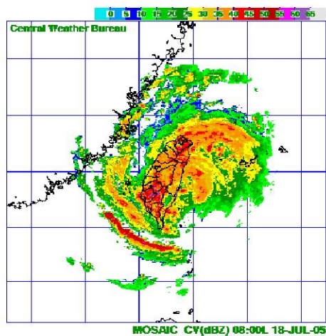
圖 12c. 同圖 12a, 但為 94 年 7 月 18 日 8 時(地方時) Fig. 12c. Same as 12a, but for 071808L 2005
