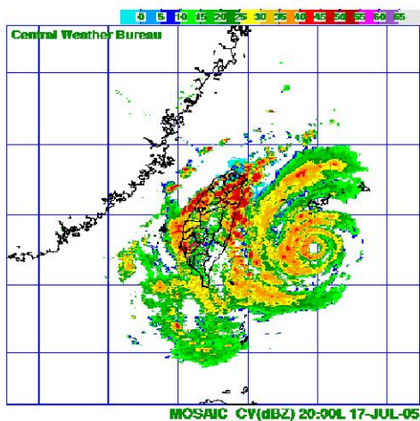
圖 12a. 94 年 7 月 17 日 20 時(地方時)雷達降水回波圖 Fig. 12a. The chart of radar echoes at 071720L 2005
