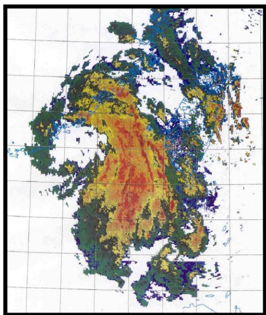
圖 7. 2005 年 8 月 13 日 0100 UTC 中央氣象局雷達網所觀測之回波圖。
