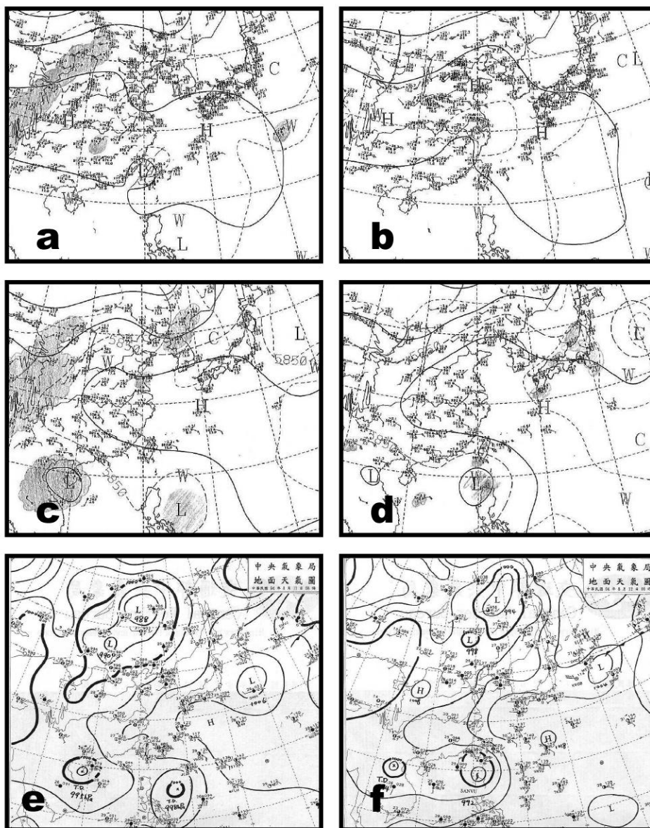
圖 4. 2005 年 8 月(a) 11 日 0000 UTC 之 300 hPa 高空分析圖，(b) 12 日 0000 UTC 之 300 hPa 高空分析圖，(c) 11 日 0000 UTC 之 500 hPa 高空分析圖，(d) 12 日 0000 UTC 之 500 hPa 高空分析圖，(e) 11 日 0000 UTC 之地面分析圖，(f) 12 日 0000 UTC 之地面分析圖。
