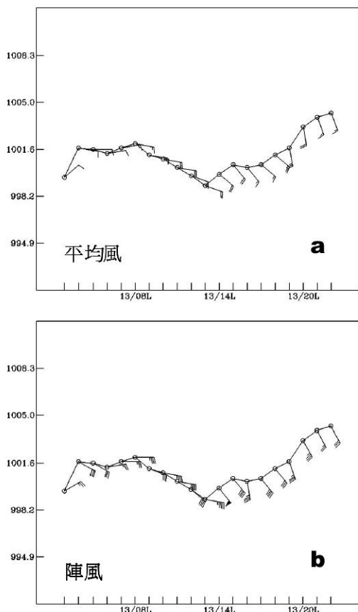
圖 8. 2005 年 8 月 13 日 3 時至 22 時 (地方時) 金門 (46711) 站 (a) 逐時平均風 及 (b) 逐時陣風與海平面氣壓之時間序列
