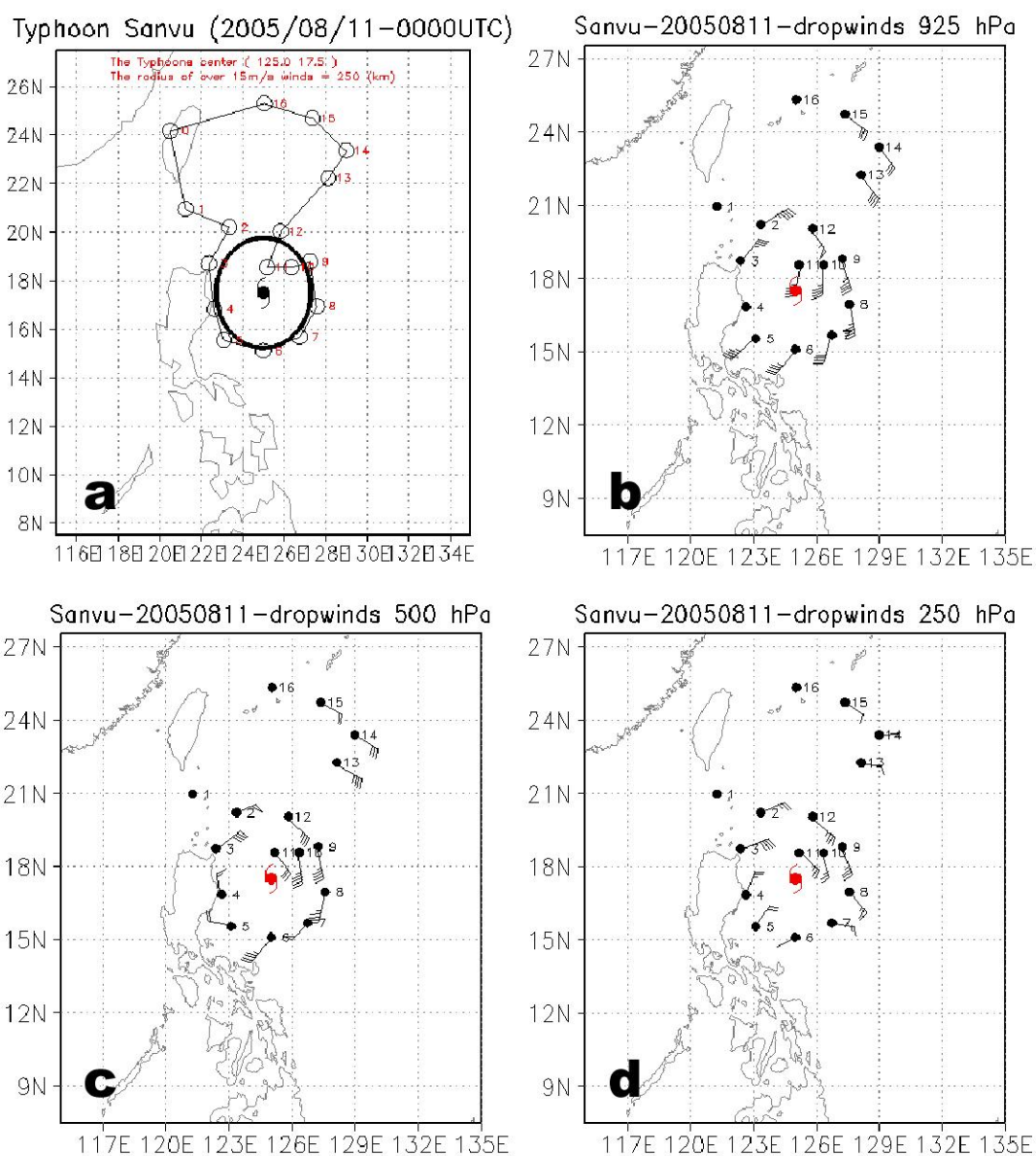
圖 6. 珊瑚颱風 GPS dropwindsonde 之(a) 觀測路徑及(b) 925 hPa (c)500 hPa (d)250 hPa 觀測風場資料 (摘自台灣大學大氣科學研究所吳俊傑教授網站)。
