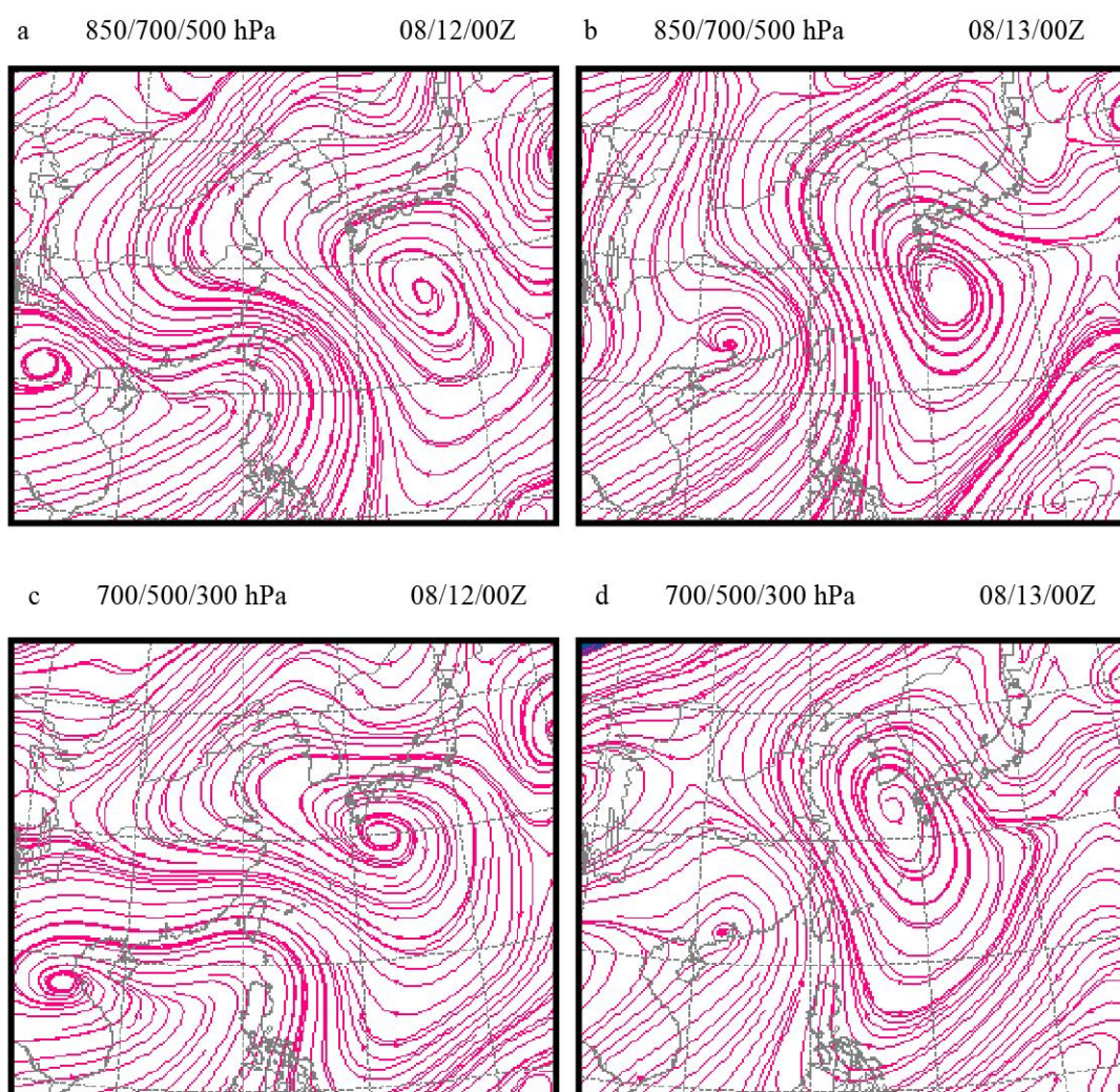
圖 5. 2005 年 8 月(a) 12 日 0000 UTC 之 850/700/500 hPa 平均氣流圖，(b) 13 日 0000 UTC 之 850/700/500 hPa 平均氣流圖，(c) 12 日 0000 UTC 之 700/500/300 hPa 平均氣流圖與 (d) 13 日 0000 UTC 之 700/500/300 hPa 平均氣流圖。 Fig. 5. The 850/700/500 hPa mean flow streamlines at (a) 0000 UTC 12, (b) 0000 UTC 13 August 2005 and the 700/500/300 hPa mean flow streamlines at (c) 0000 UTC 12, (d) 0000 UTC 13 August 2005.
