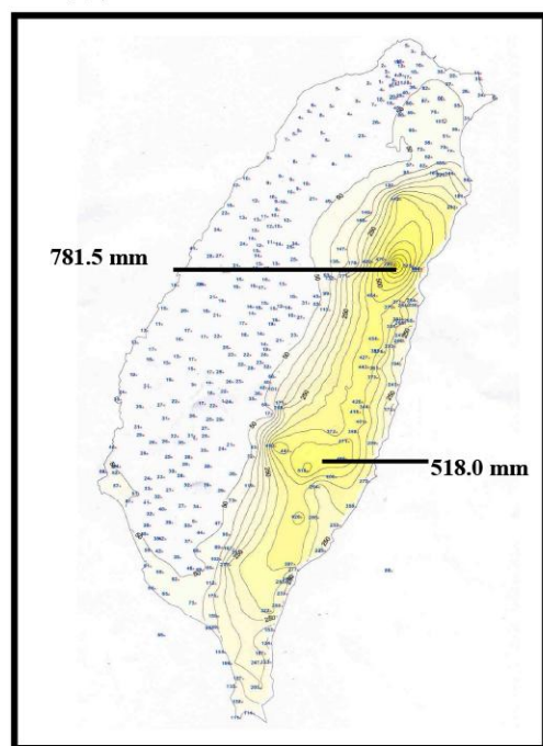
圖 9. 2005 年第 10 號颱風珊瑚等雨量線圖 (自 8 月 10 日 1600 UTC 至 8 月 13 日 1200 UTC 止)
