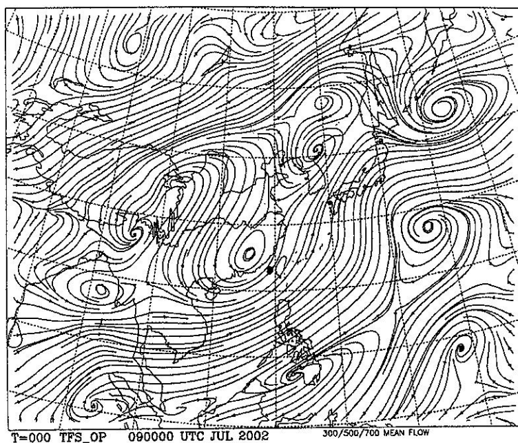
圖 4b：2002 年 7 月 9 日 0000UTC 300/500/700 百帕平均氣流圖。
