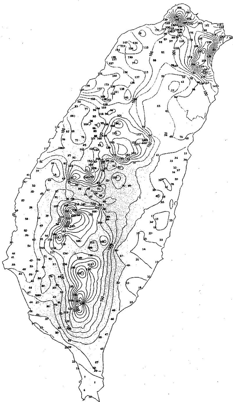
娜克莉颱風雨量分布圖
