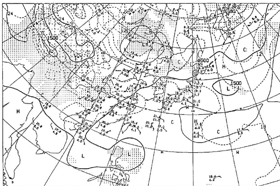
圖 1b. 8 月 3 日 0000UTC 850hPa 和 700hPa 高空天氣圖
