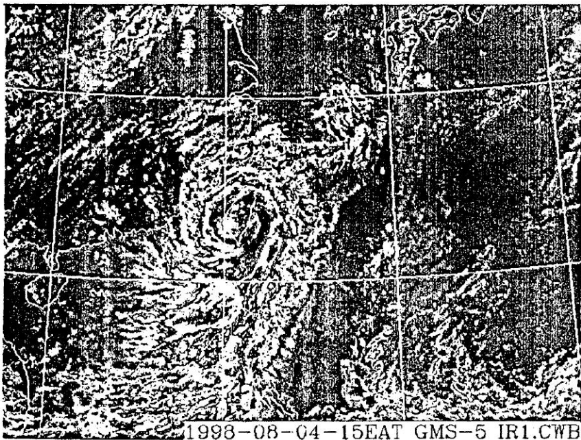
圖 3d. 1998 年 8 月 4 日 15 時紅外線雲圖，奧托颱風正在台灣陸地上
