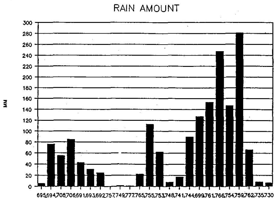
圖 9. 艾美颱風過境期間，氣象局各測站的總雨量圖
