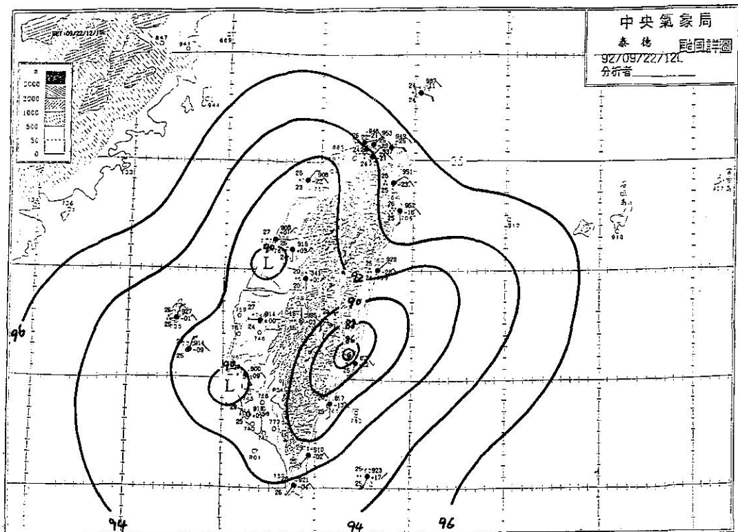
圖8 泰德颱風地面詳圖分析 (登陸時) Fig.8 : Mesoanalysis surface chart of tropical storm 「TED」.
