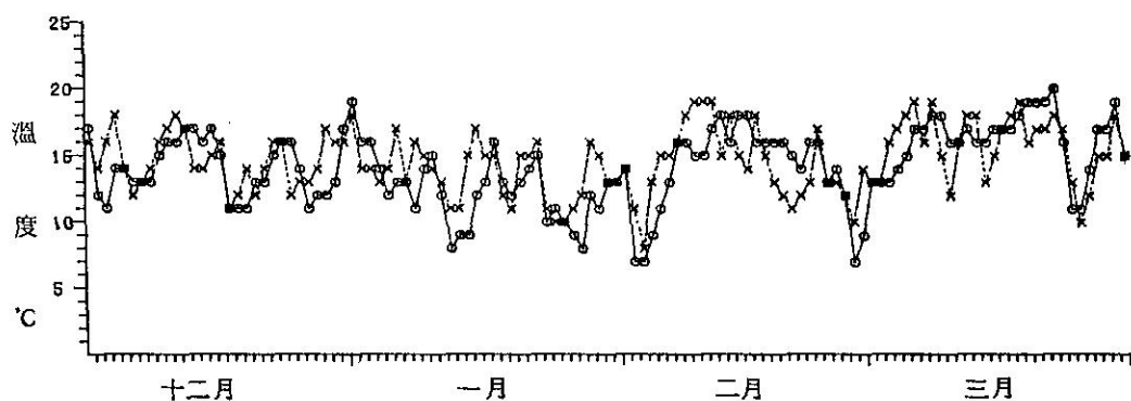
圖五 東北部地區12小時預報(x)與逐日實際觀測最低溫度(o)之相對分佈
