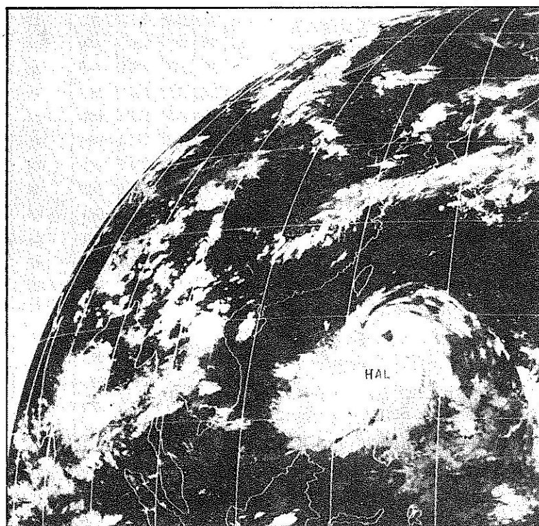
圖二、 海爾颱風衛星雲圖 (74年6月21日 12Z GMS 衛星所攝)
