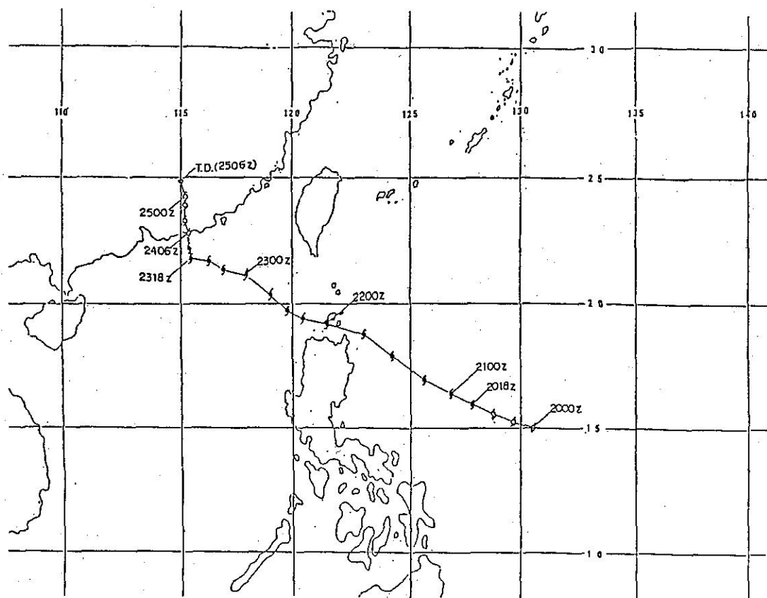
圖五、海爾颱風之最佳路徑圖（6月20日 00Z 至 6月25日 06Z）
