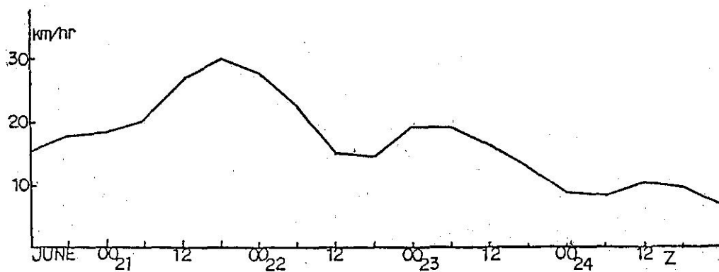
圖六、海爾颱風之移動速率變化曲線（6月20日 00Z 至 6月25日 00Z）
