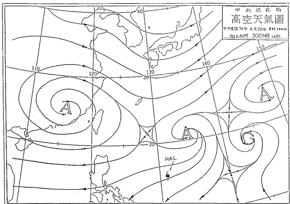
圖一、 74年6月20日 00Z 300 mb 氣流線圖
