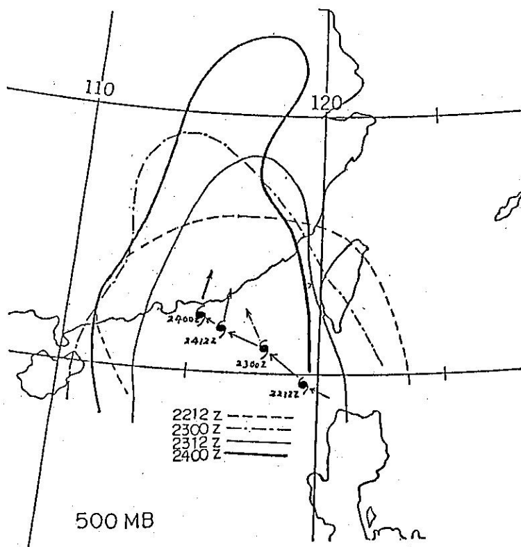
圖十一、500mb 24小時最大高度下降區與颱風路徑圖
