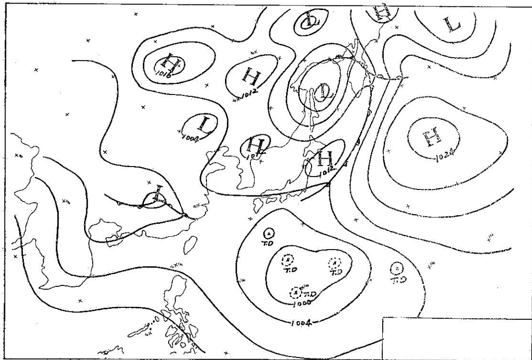
Fig 2. Sea level synoptic chart. COCOZ 14h. Aug. 1977. 圖 2. 66年 8月 14日 8時地面圖
