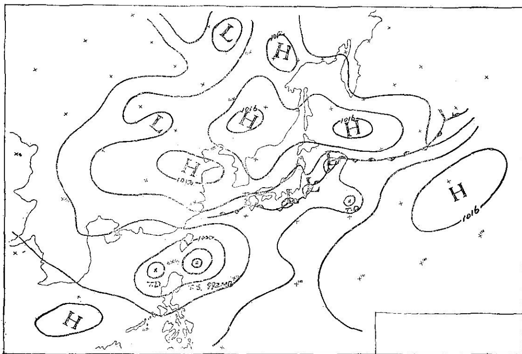
圖 4. 66年8月19日20時地面圖
