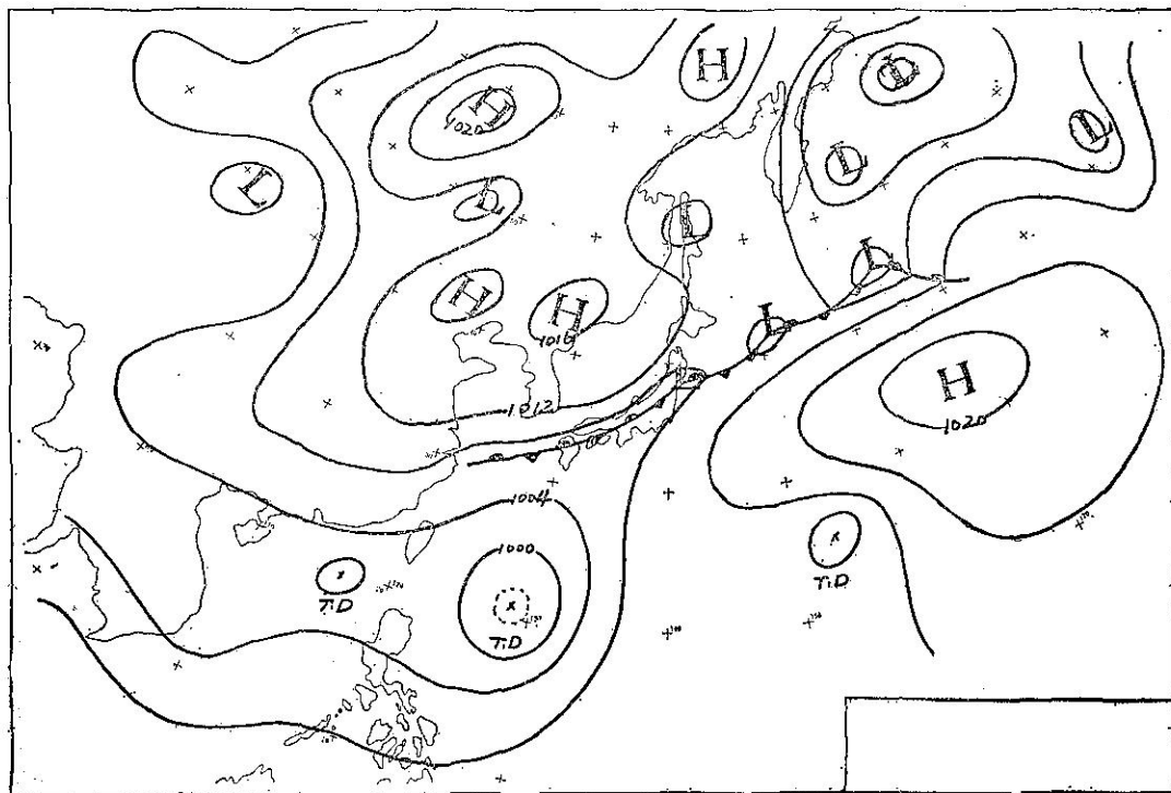
圖 3. 66年8月18日8時地面圖
