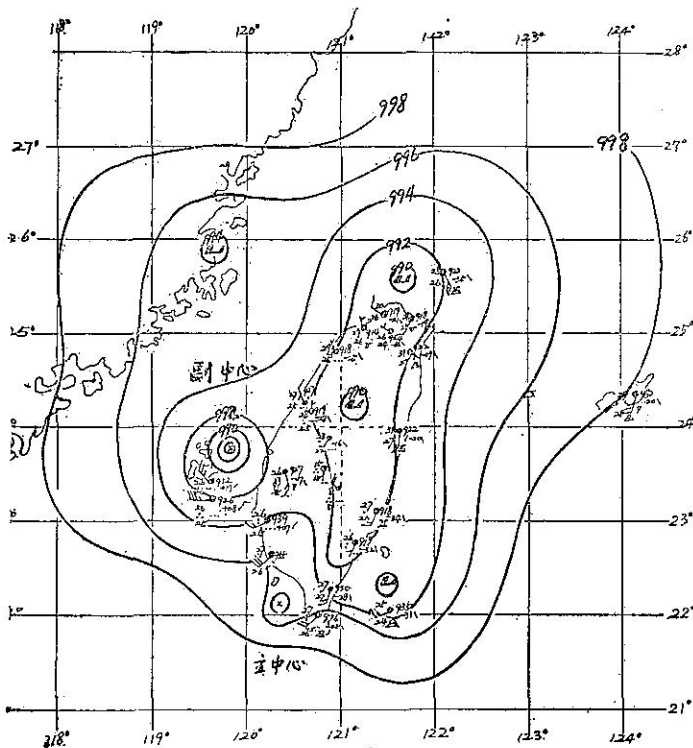
圖 5 a. 民國 66 年 8 月 22 日 14 時 颶風圖
