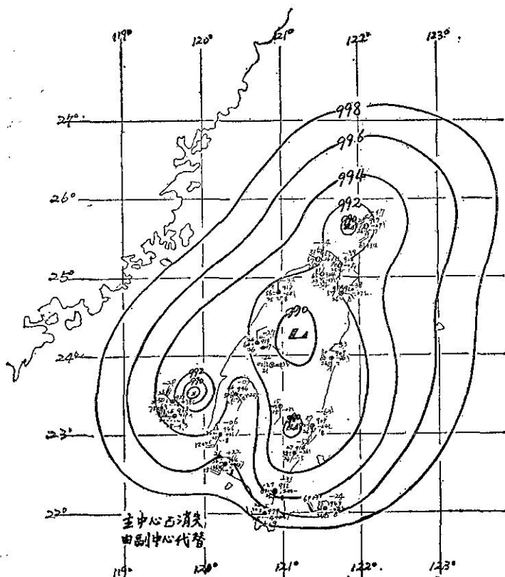
圖 5 b. 民國 66 年 8 月 22 日 15 時 颱風圖
