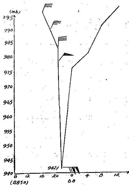
圖6：宜蘭最低氣壓與最大風速變化圖
