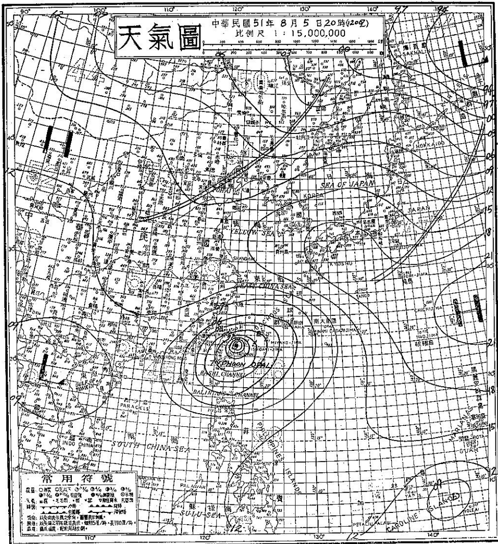
圖 4：歐珀颱風即將登陸時 700mb 高空圖
