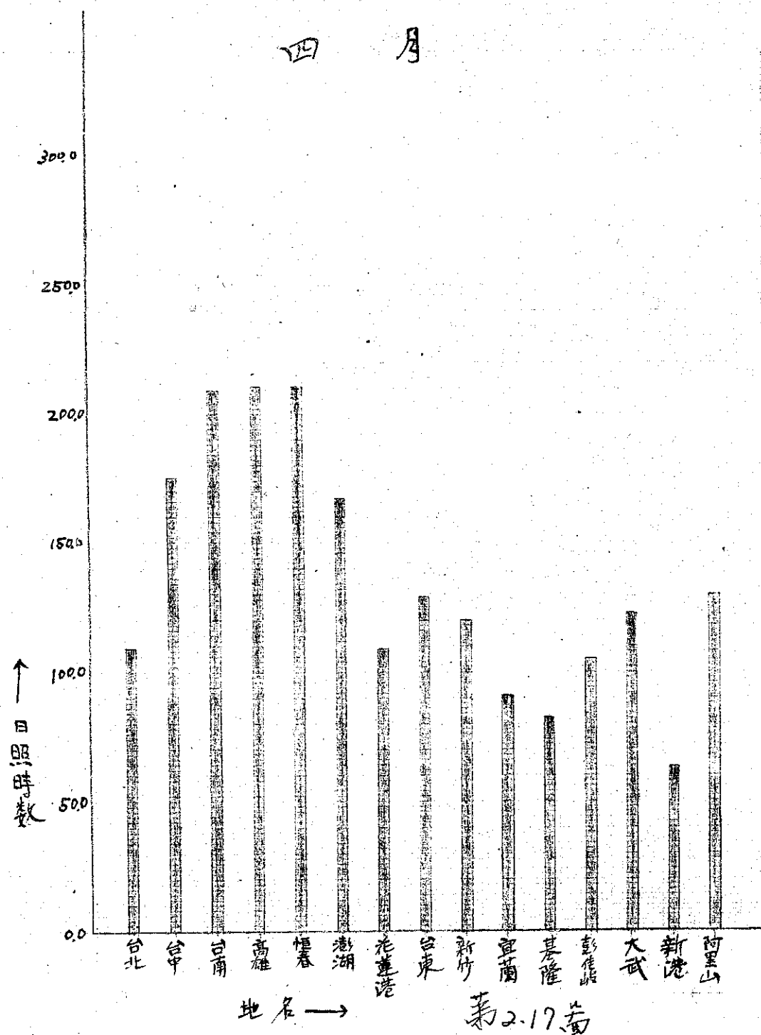
各年度各月平均日照時數比較圖表
