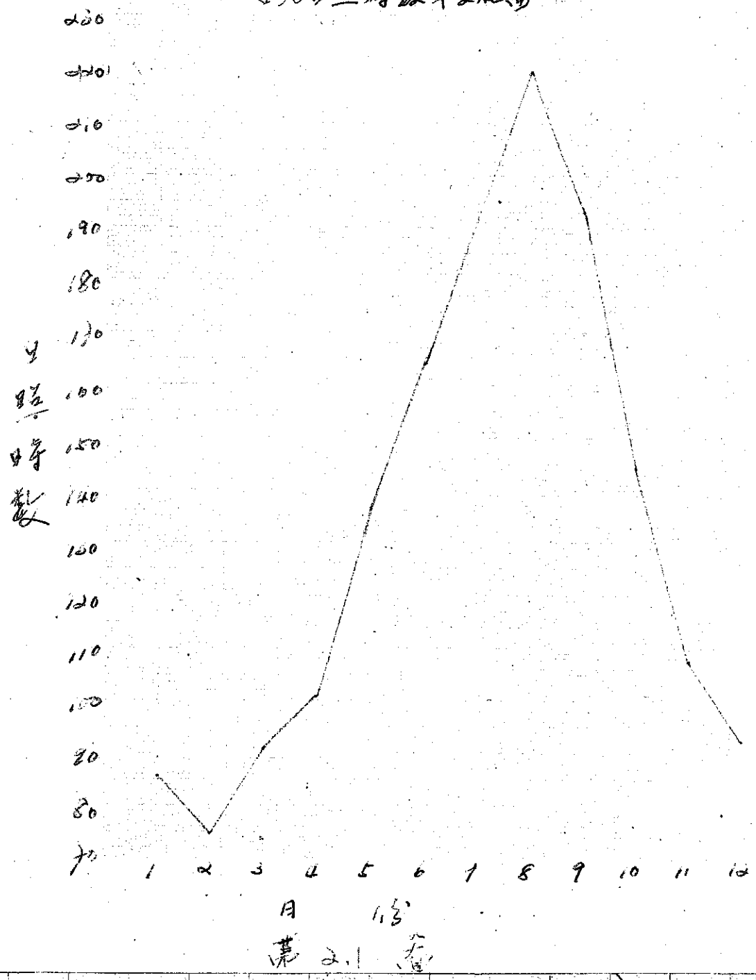
台北日照時數年變化圖
