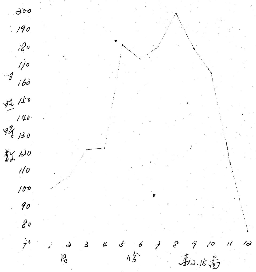
大武日照時數年變化圖
