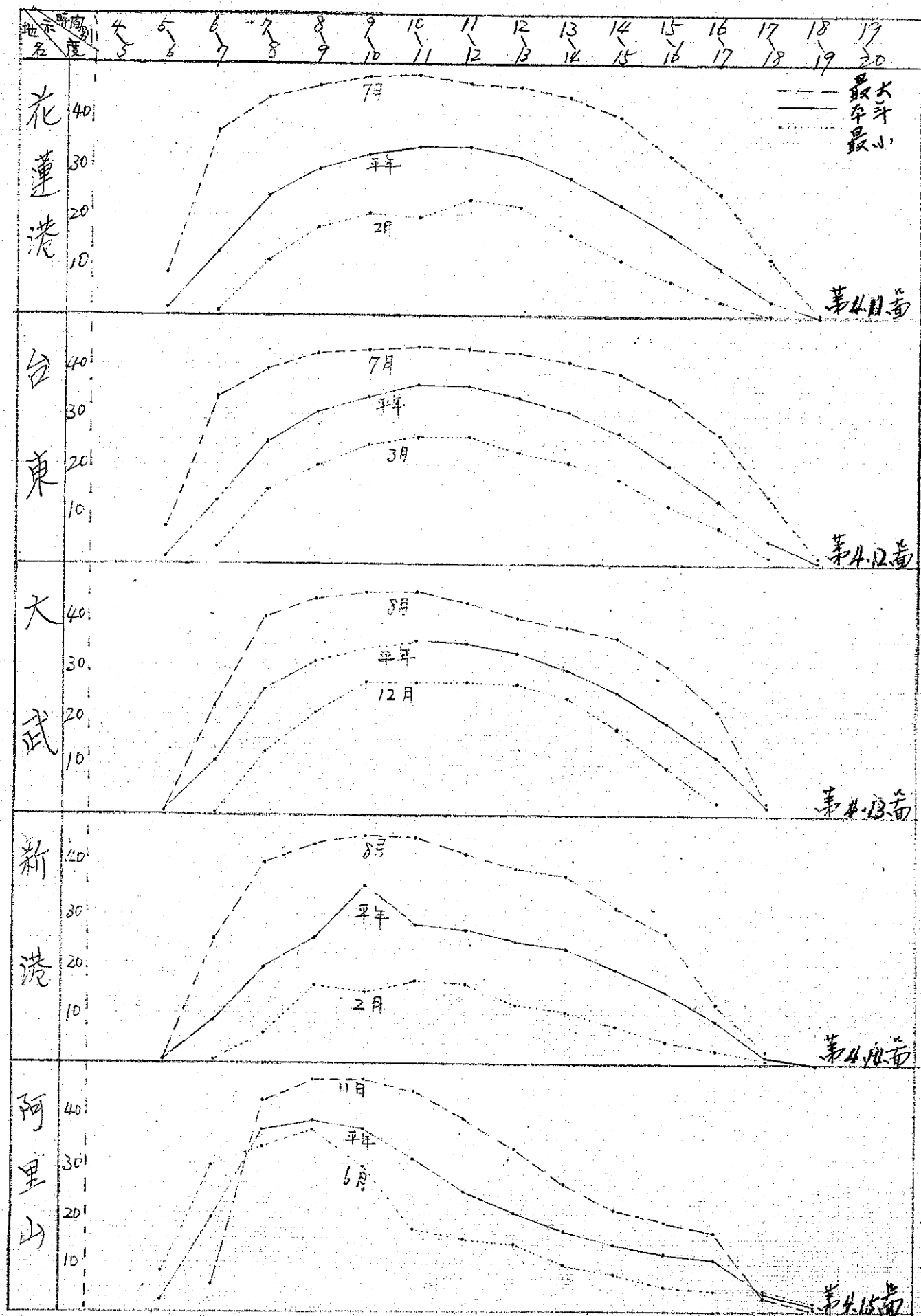
各地常年平均時別日照時數比較圖表
