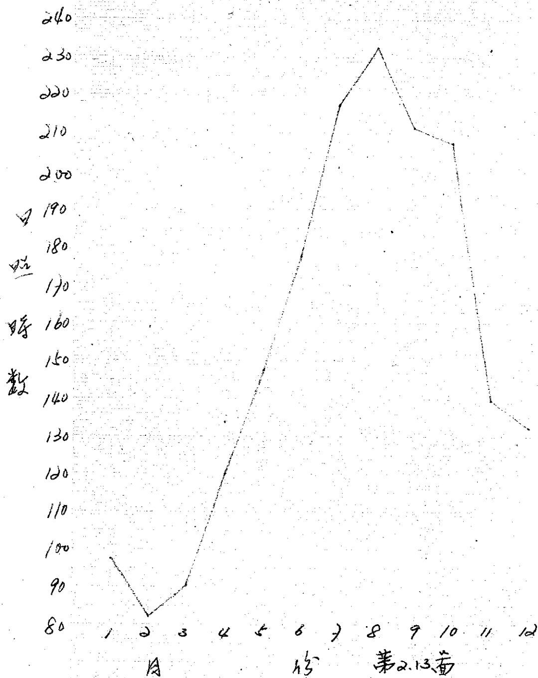
新竹日晷時數年變化圖
