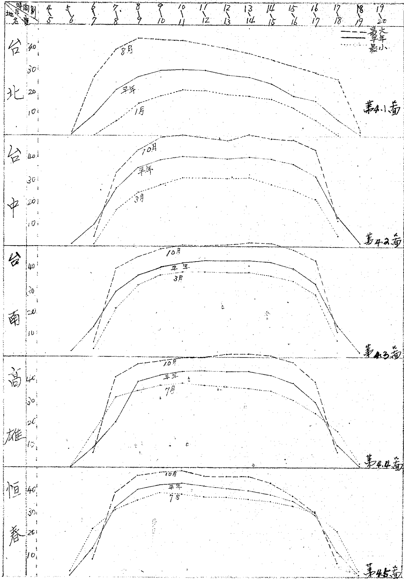
各地累年平均時制日照時數比較圖表
