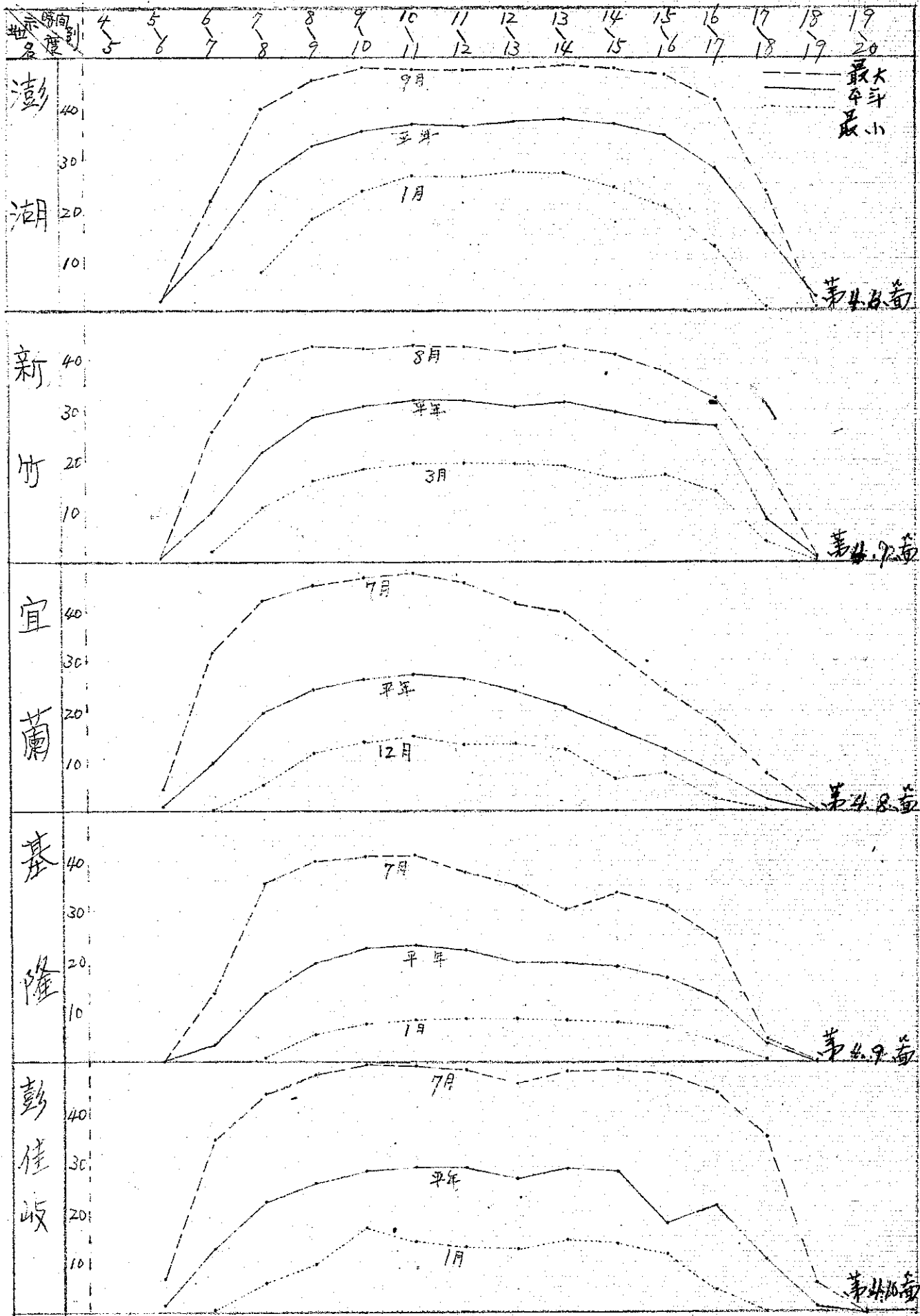
各地年平均日照時數比較圖表
