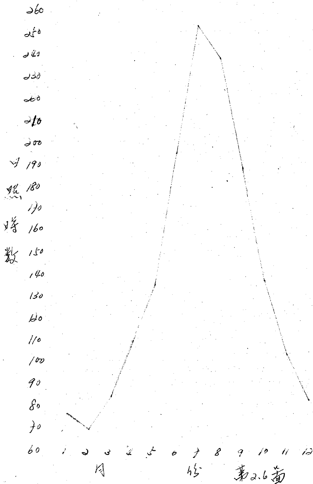
花蓮港日照時數年變化圖
