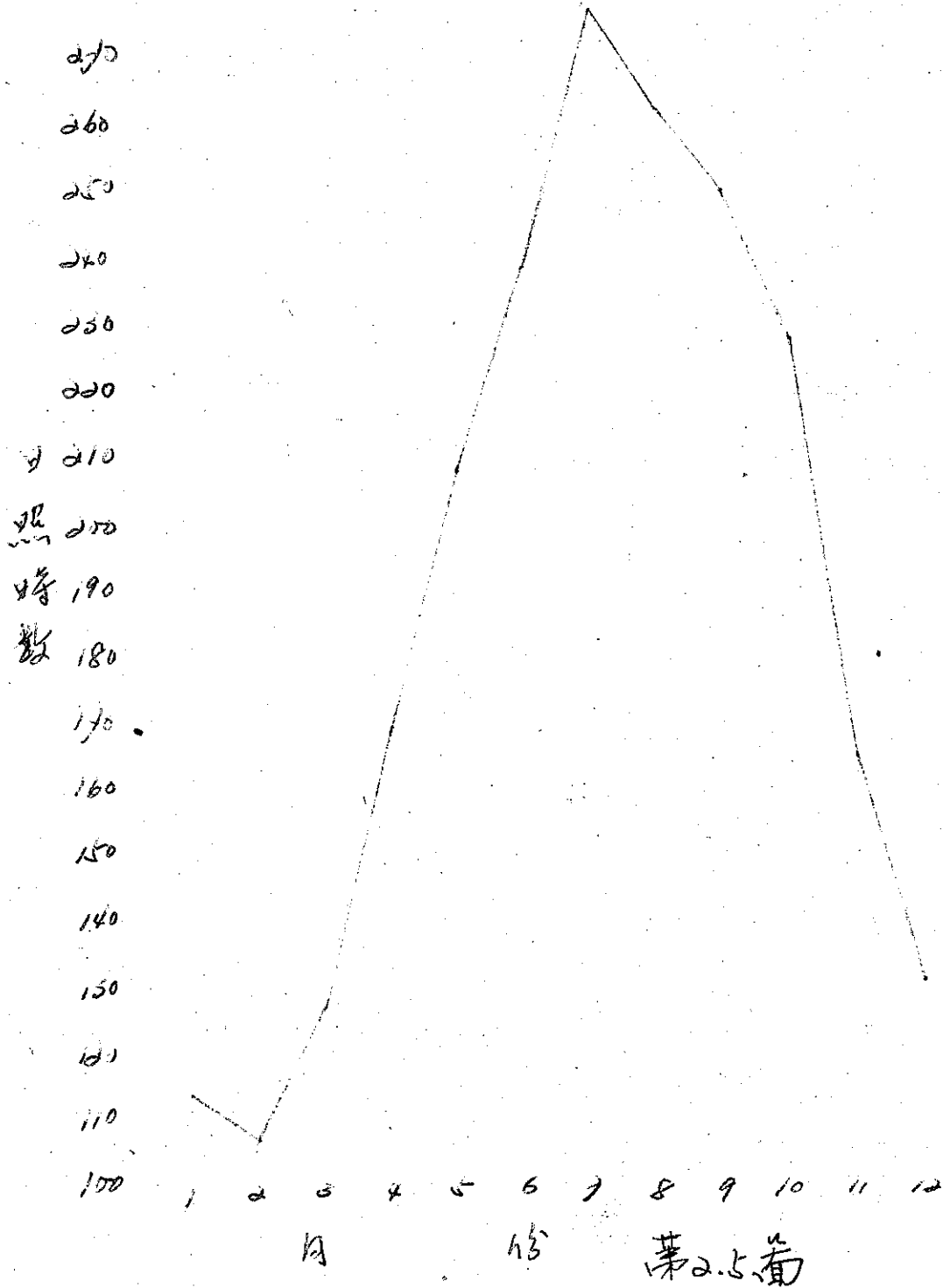
澎湖日照時數年變化圖
