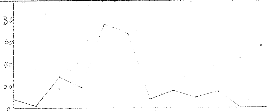
彭佳嶼累年平均雷雨降雨量圖表
