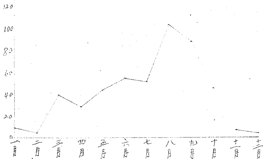
澎湖累年平均雷雨降雨量圖表
