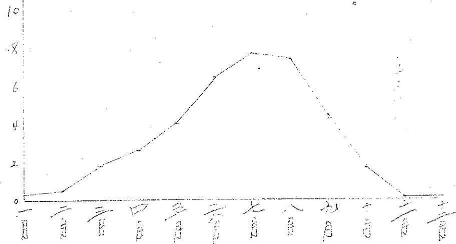
全省常年平均雷雨回数圖表
