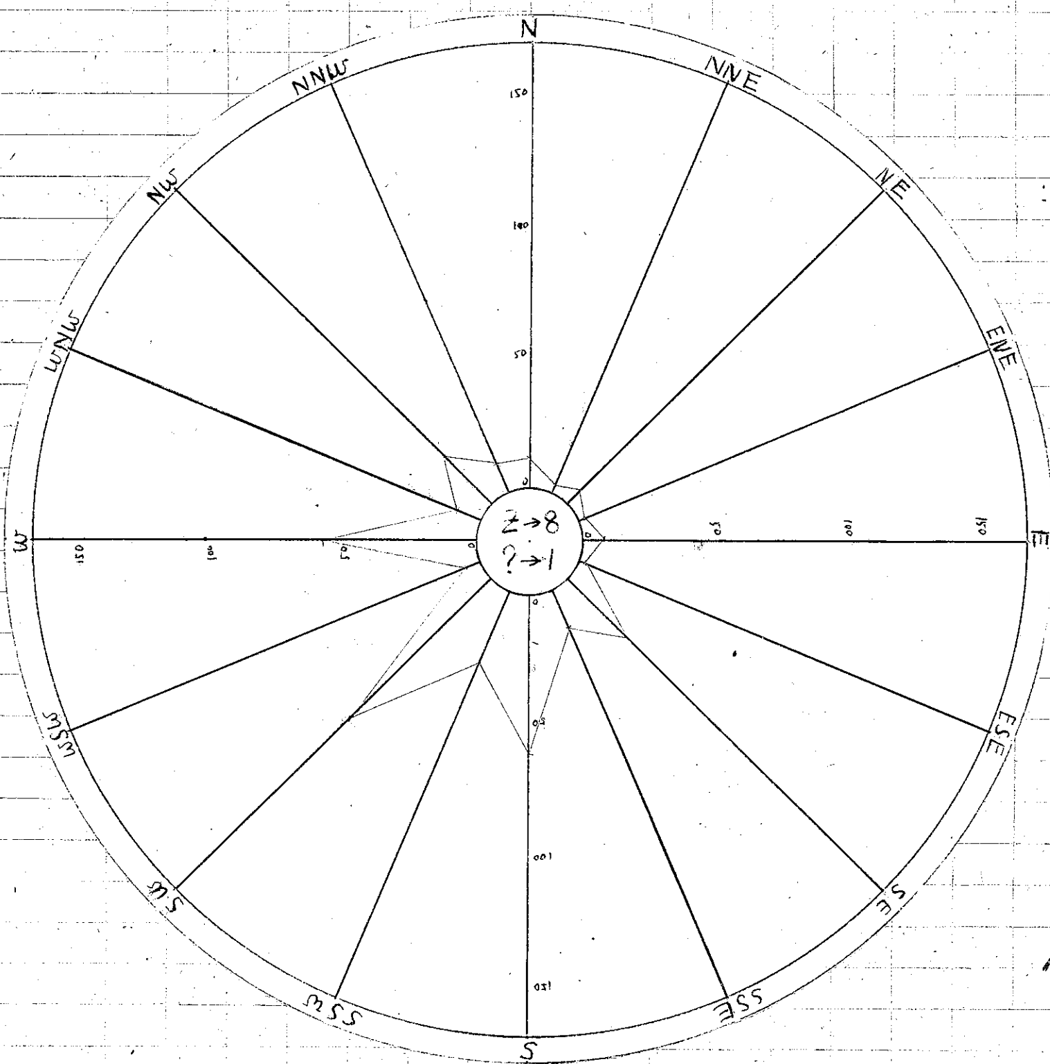
彭佳屿雷雨方向别发生回数统计表
