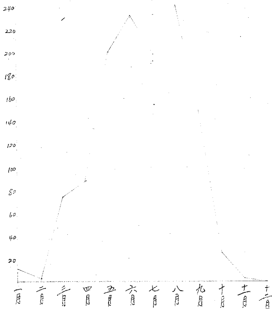
阿里山累年平均雷雨降雨量圖表
