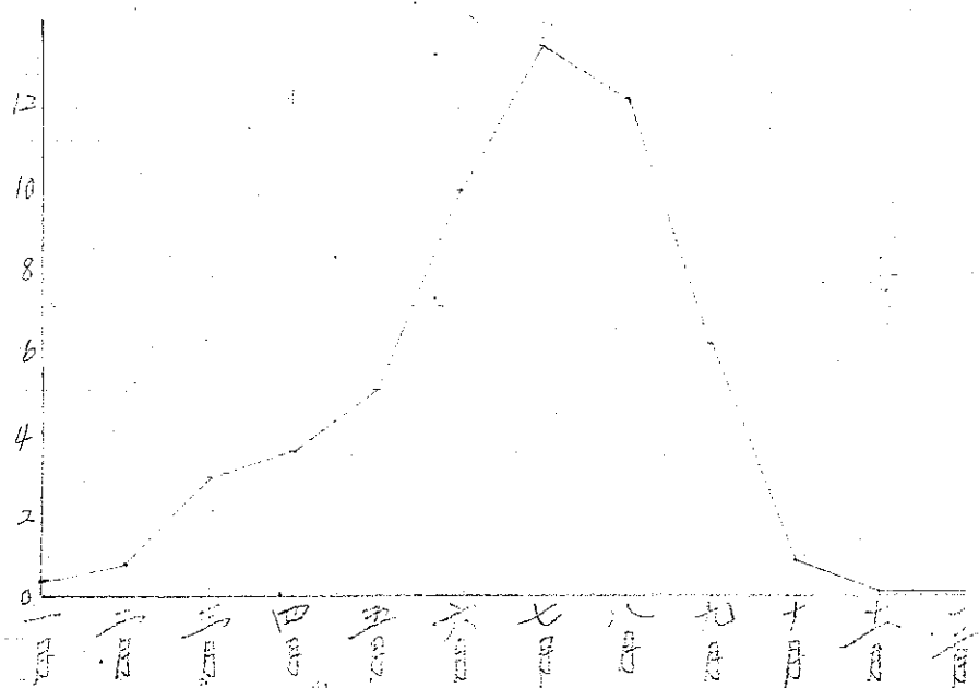
台中年平均雷雨回数圖表
