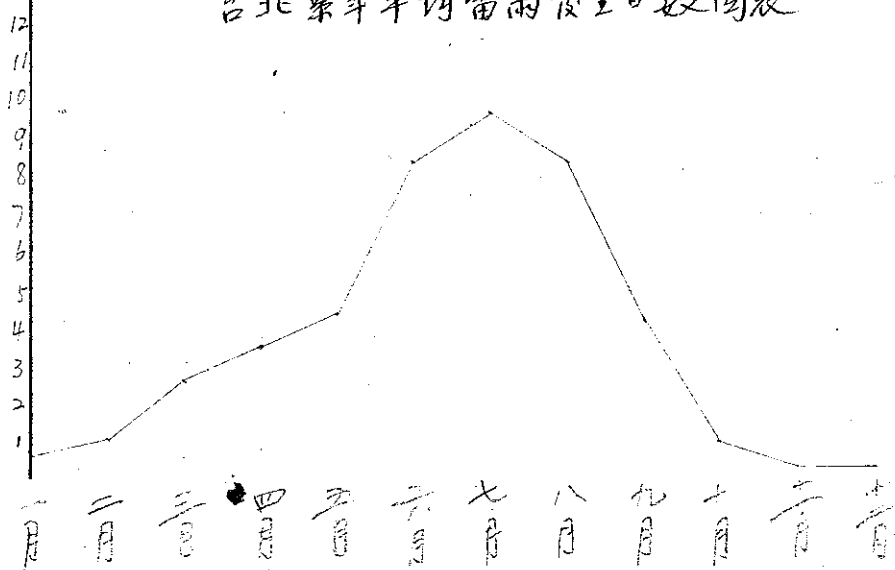
台北累年平均雷雨發生日數圖表
