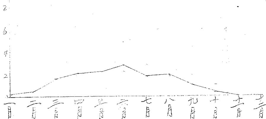
彭佳嶼年平均雷雨回数圖表
