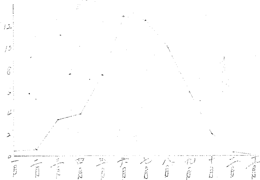
宜蘭單年平均雷雨回數圖表
