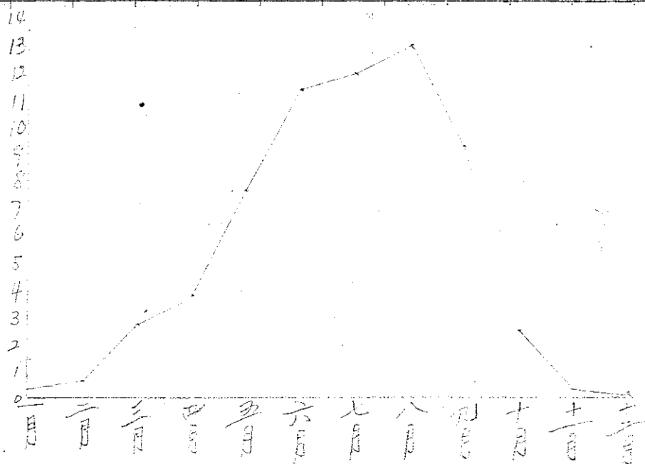
阿里山羣年平均雷雨回数圖表
