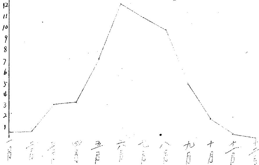
宜蘭累年平均雷雨發生日數圖表
