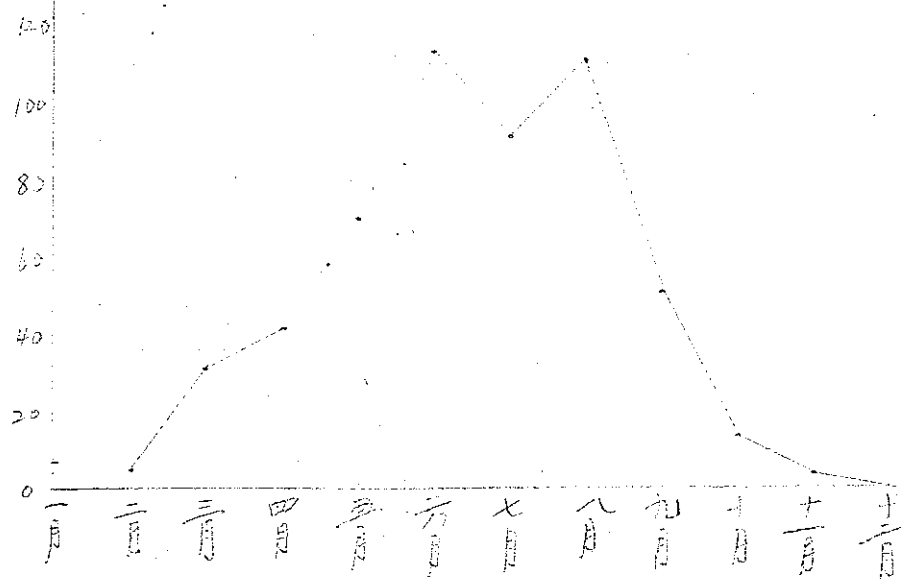
全省累年總平均雷雨降雨量圖表
