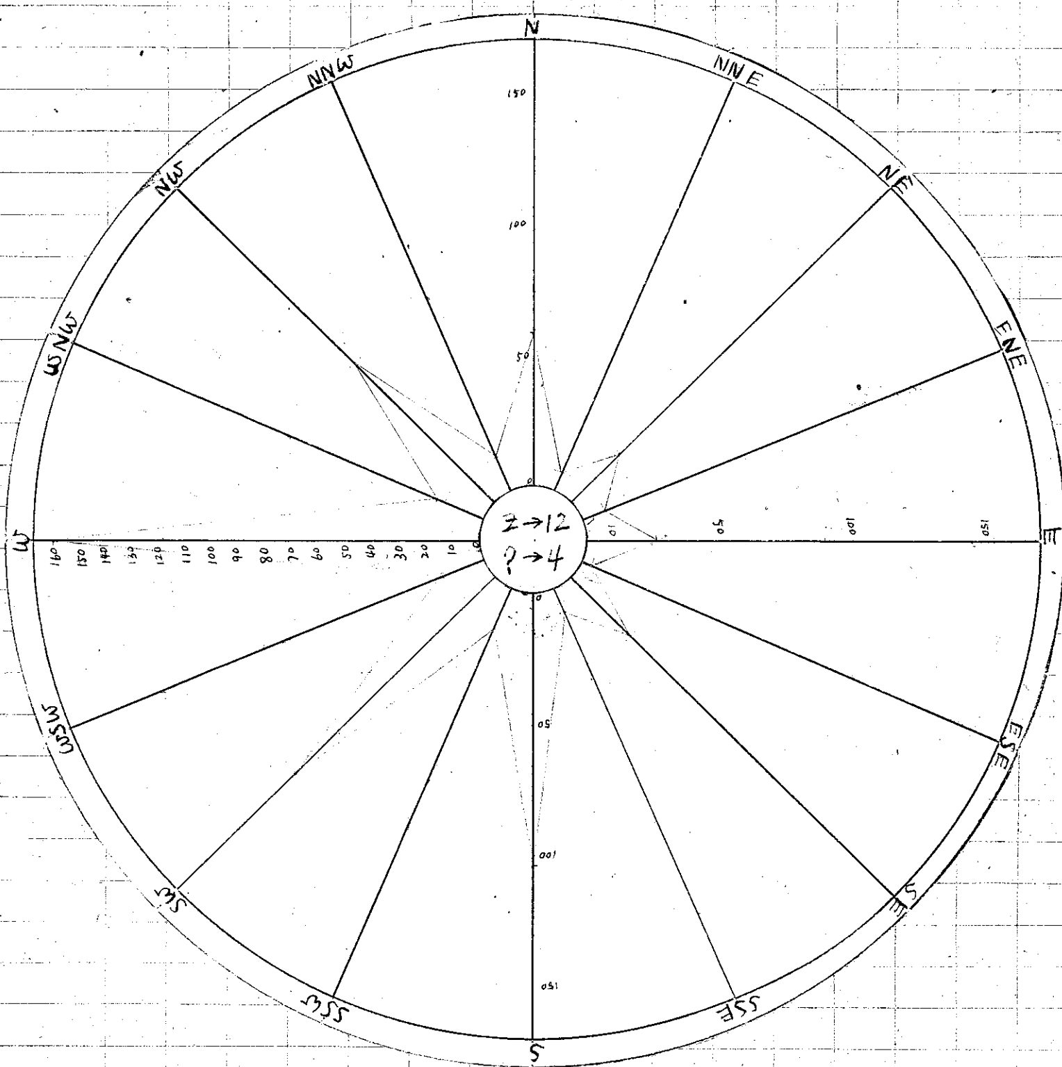
阿里山雷雨方向别发生回数统计表
