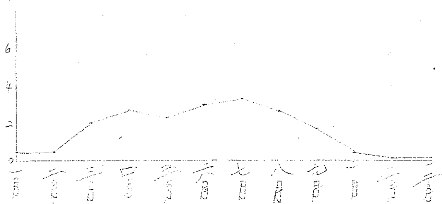
澎湖羣年平均雷雨回数圖表
