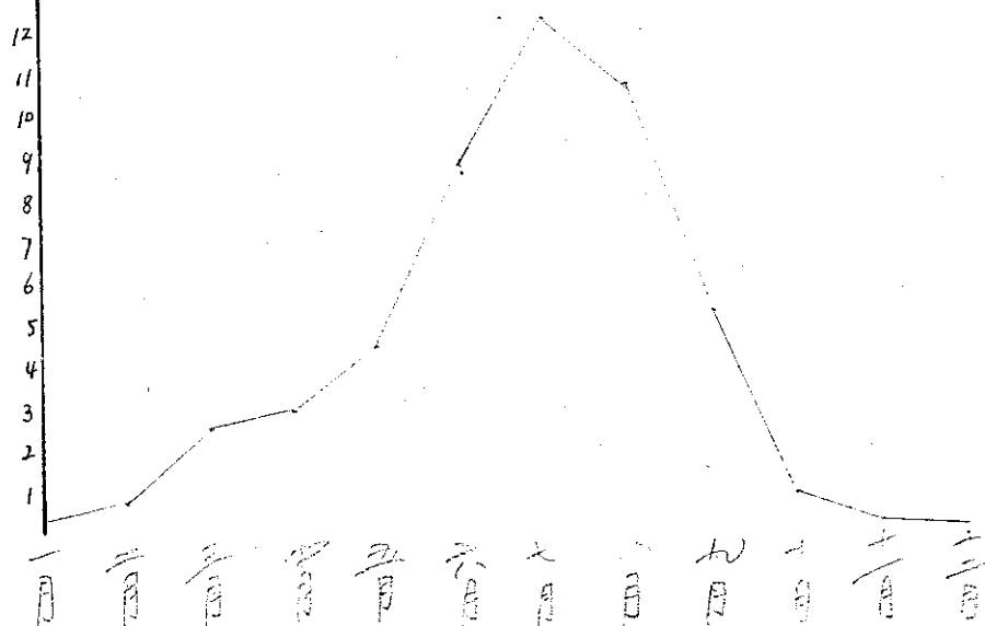
台中累年平均雷雨發生日數圖表
