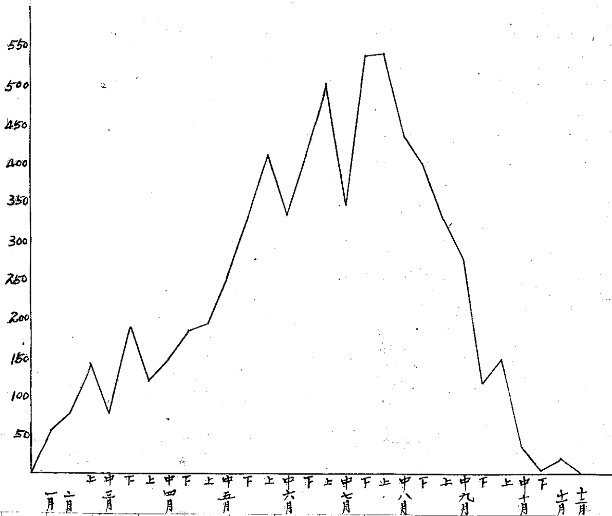
台灣全省十年間旬別雷雨發生回數統計表
