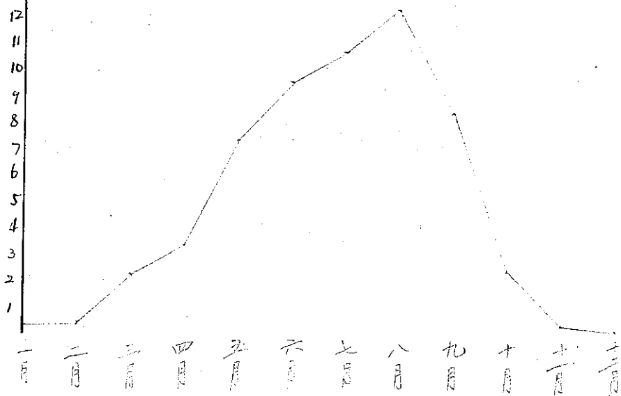
阿里山累年平均雷雨發生日數圖表
