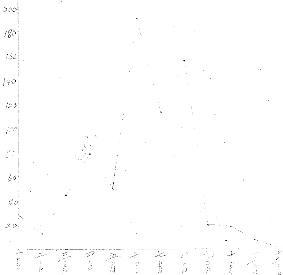
台北累年平均雷雨降雨量圖表
