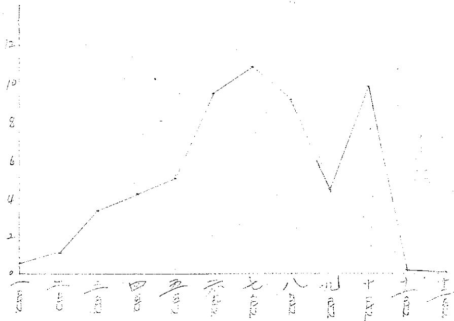
台北常年平均雷雨回数圖表
