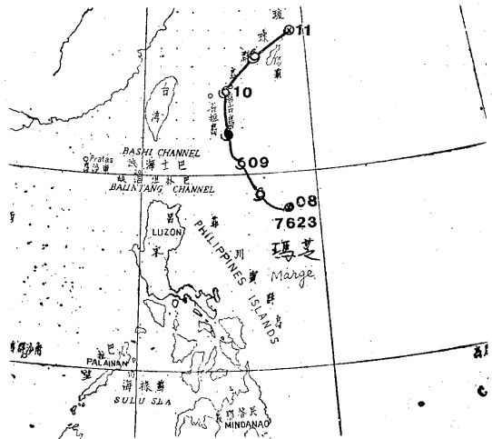
圖 13. 民國 65 年 11 月份颱風路徑圖 Fig. 13. Typhoon tracks in November, 1976.
