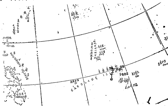
圖5. 民國65年2月份颱風路徑圖 Fig. 5. Typhoon tracks in February, 1976.
