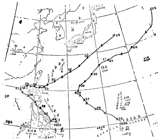
圖 8. 民國 65 年 6 月份颱風路徑圖 Fig. 8. Typhoon tracks in June, 1976.
