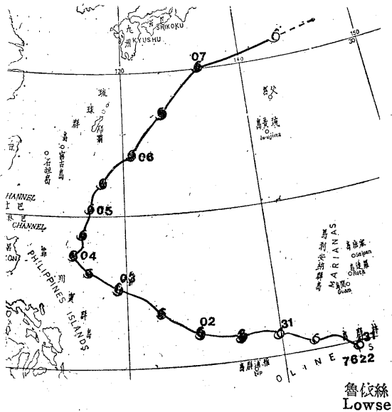
圖 12. 民國 65 年 10 月份颱風路徑圖 Fig. 12. Typhoon tracks in October, 1976.
