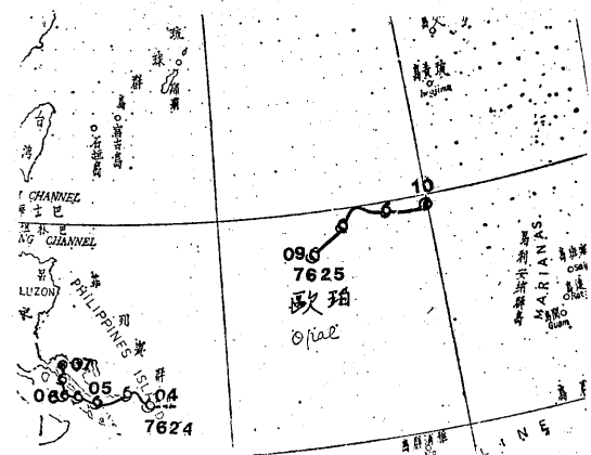
圖 14. 民國 65 年 12 月份颱風路徑圖 Fig. 14. Typhoon tracks in December, 1976
