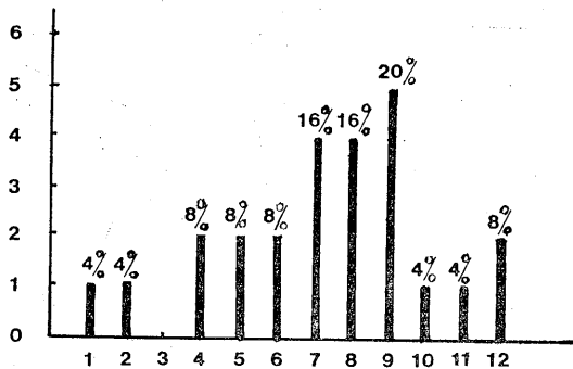
圖 1 民國 65 年北太平洋西部所發生颱風之逐月分配及其百分比
