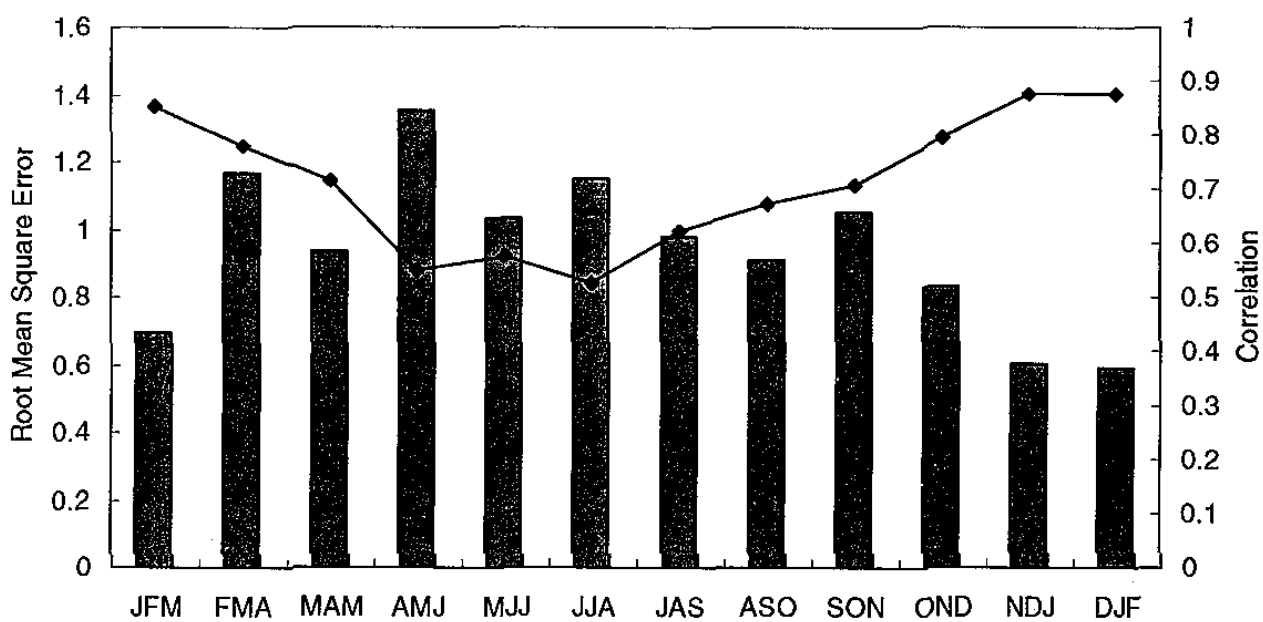
圖 3、Niño3.4 lead2 預報之均方根誤差（長條圖）及相關係數（折線圖）。
