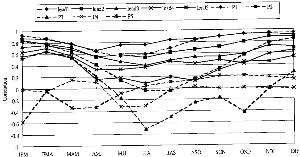
圖 2、Niño3.4 模式預報及持續法之交叉驗證。其中 lead1 表示領先 1 季之正準相關分析法，P1 表示領先 1 季之持續法……以此類推。
