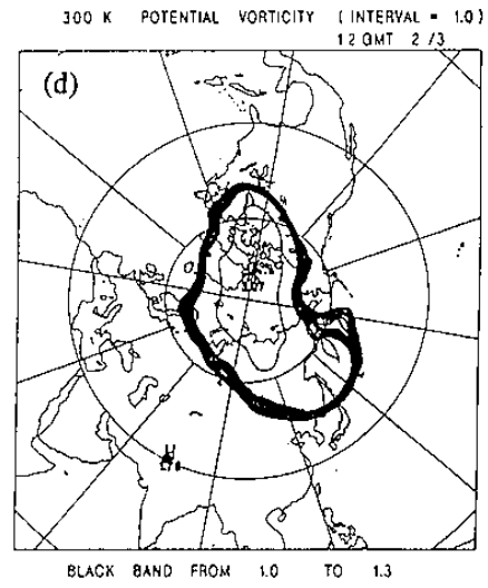
圖7：暖冬年300 0 K等熵面位渦分佈圖，圖中之寬黑線帶為位渦值在1.0~1.3Ps之區間。(a) 11月，(b) 12月，(c) 1月，(d) 2月。
