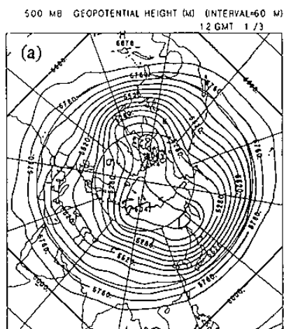
圖4：500 百帕面一月份高度場合成圖。(a) 暖冬年，(b) 冷冬年。
