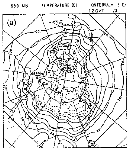
圖3：950 百帕面一月份平均氣溫之合成圖。(a) 暖冬年，(b) 冷冬年。
