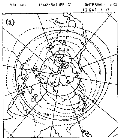
圖2：500 百帕面一月份平均氣溫之合成圖。(a) 暖冬年，(b) 冷冬年。
