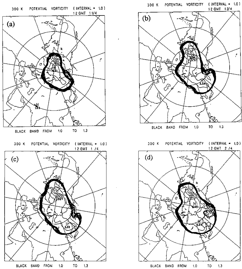
圖9：冷冬年300 0 K等熵面位渦分佈圖，圖中之寬黑線帶為位渦值在1.0~1.3 Ps之區間。(a) 11月，(b) 12月，(c) 1月，(d) 2月。
