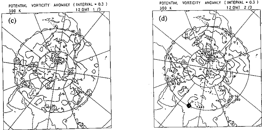
圖8：暖冬年300 0 K等熵面位渦距平分佈圖，等值線間距為0.3 Ps。 (a) 11月，(b) 12月，(c) 1月，(d) 2月。
