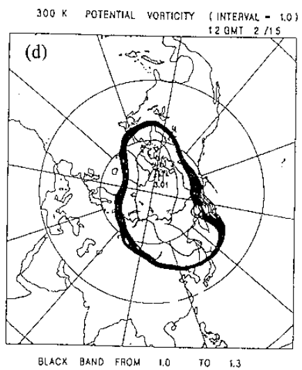
圖6：15年平均300°K等熵面位渦分佈圖，圖中之寬黑線帶為位渦值在1.0~1.3 Ps之區間。(a) 11月，(b) 12月，(c) 1月，(d) 2月。
