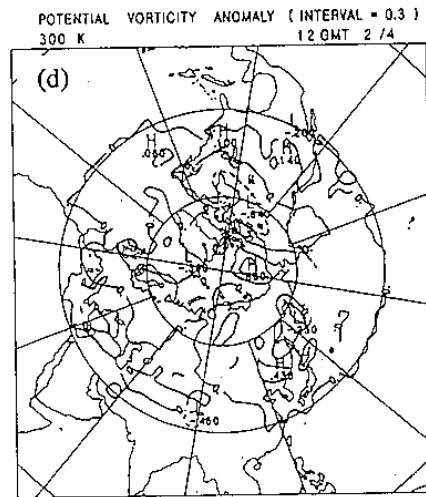
圖10：冷冬年300 0 K等熵面位渦距平分佈圖，等值線間距為0.3 Ps。 (a) 11月，(b) 12月，(c) 1月，(d) 2月。
