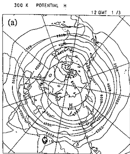
圖11：一月份300 0 K等熵面高度場分佈圖，等值線間距為1000 m。 (a) 暖冬年，(b) 冷冬年。
