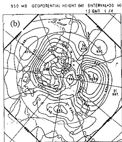
圖5：950 百帕面一月份高度場合成圖。(a) 暖冬年，(b) 冷冬年。
