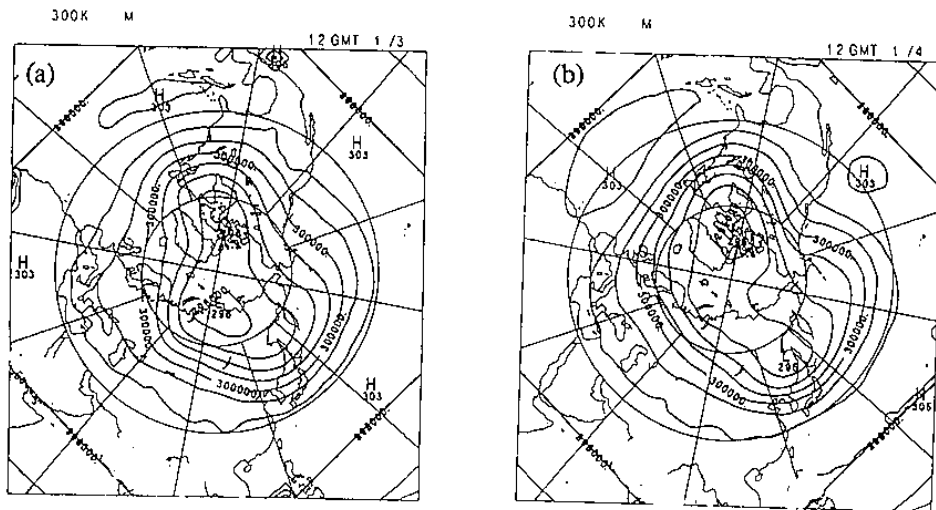
圖12：一月份300 0 K等熵面流函數場分佈圖，等值線間距為1000 m 2 sec 2 。(a)暖冬年，(b)冷冬年。
