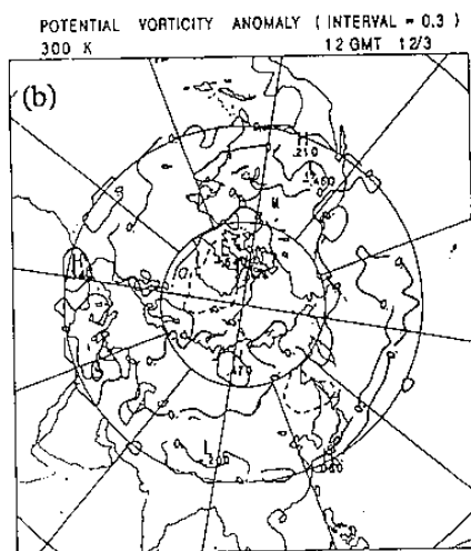
圖7：暖冬年300 0 K等熵面位渦分佈圖，圖中之寬黑線帶為位渦值在1.0~1.3Ps之區間。(a) 11月，(b) 12月，(c) 1月，(d) 2月。
