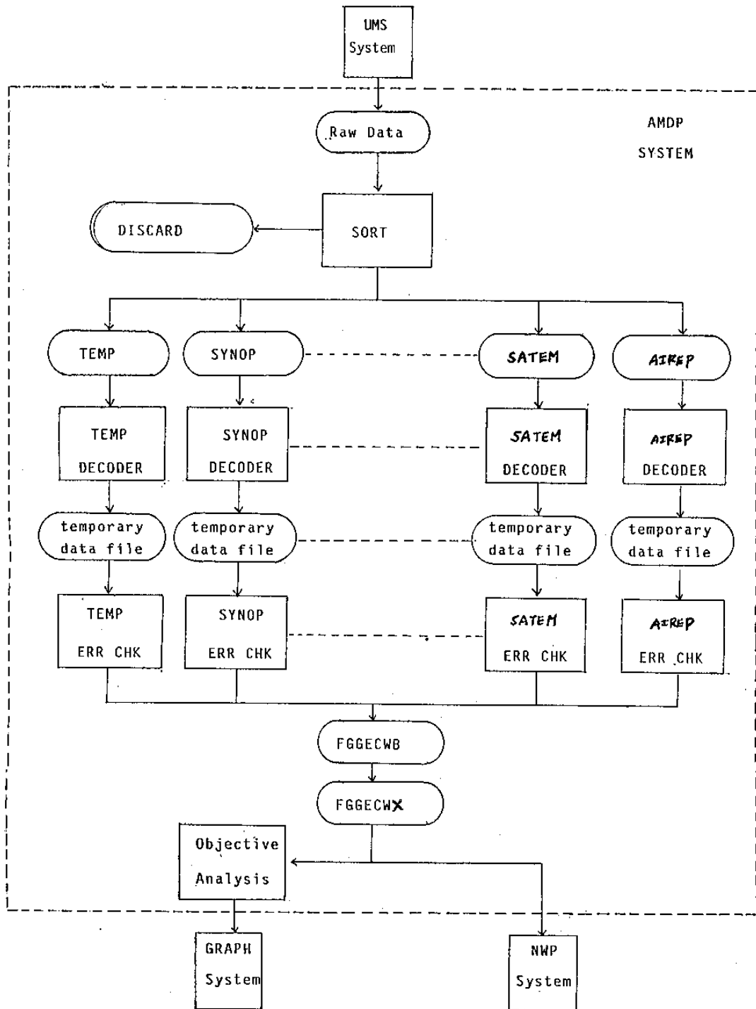
圖一 cyber 840 上 AMDP 系統架構流程。
